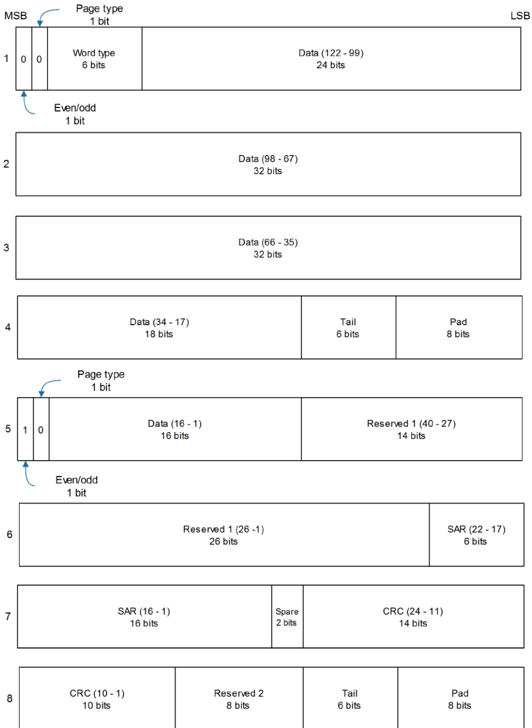
Figure 33: Galileo E1-B subframe words
